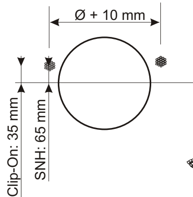
Doppelaufhängung
