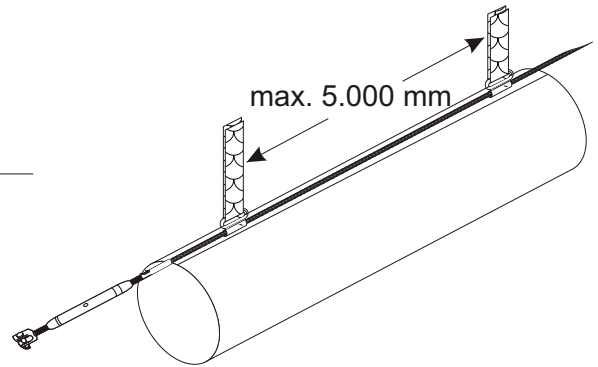
Maximalabstand Seilabhänger
